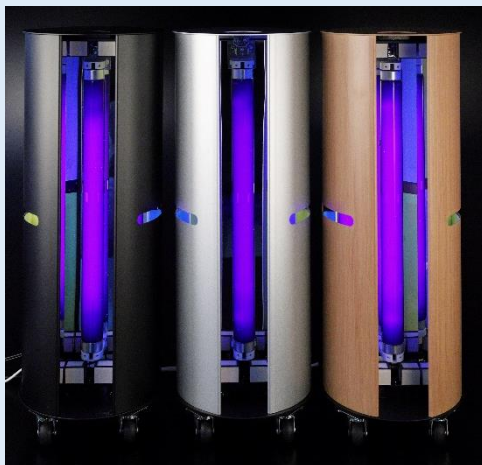
光触媒付捕虫器 トレテラ・ルミエVer.2
