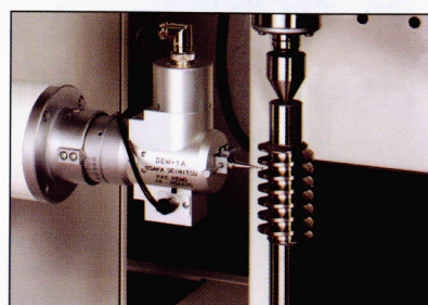
自動原点出治具 Auto zero set gauge
