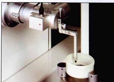
インターナルギヤ Internal gear
